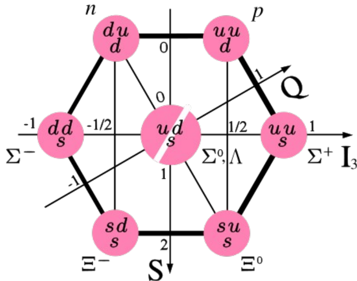
Baryon Octet
